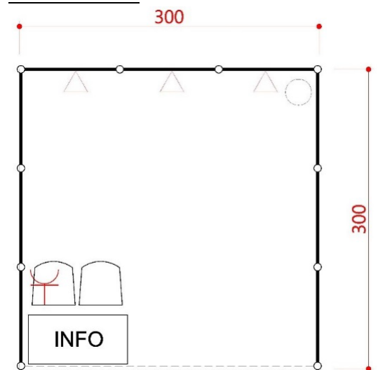
平面配置示意圖
